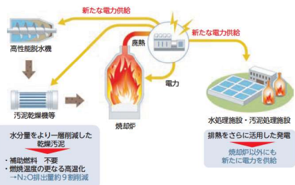
エネルギー供給型(カーボンマイナス)污泥焼却炉のイメージ
