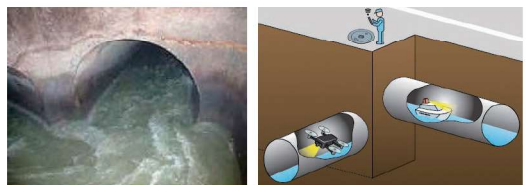
高水位の下水道管 遠隔制御による調査のイメージ
