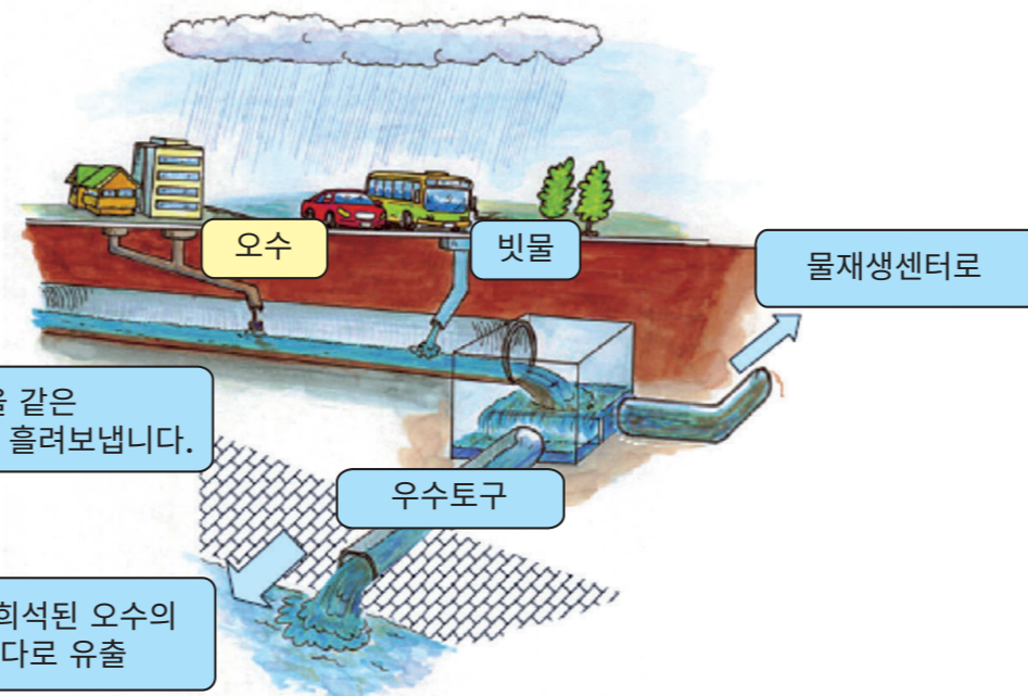
합류식 하수도의 구조 (호우 시)
