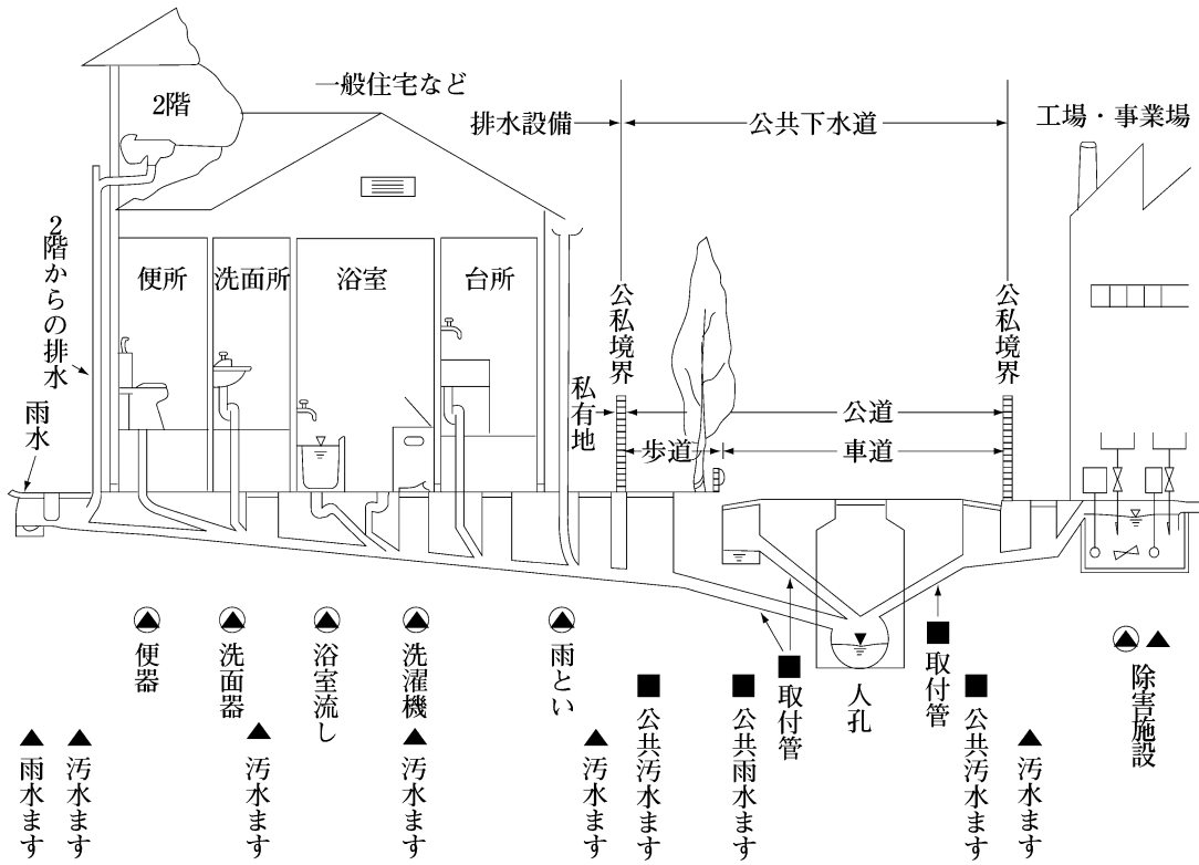
図1-1 合流式の例
