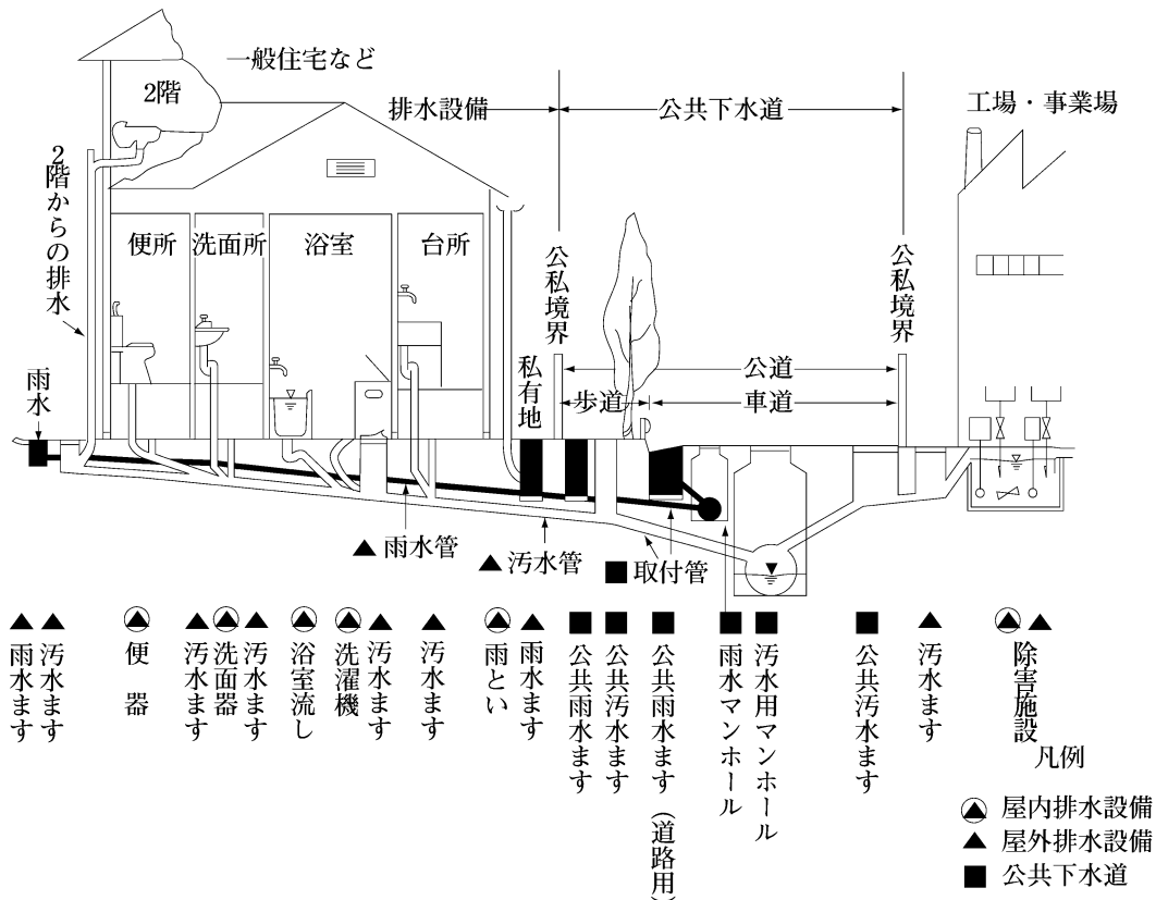
図1-2 分流式の例
