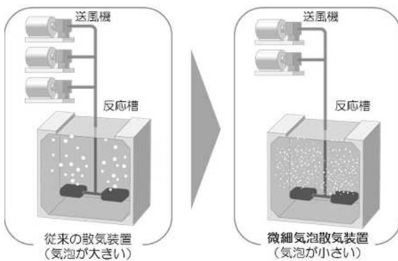
図表4-6 微細気泡散気装置のイメージ
