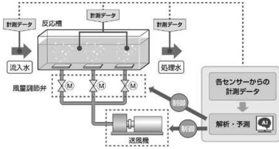
図表4-3 AIを活用した送風量制御技術のイメージ
