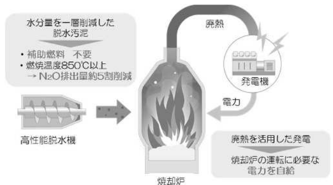
図表4-8 エネルギー自立型焼却炉のイメージ
