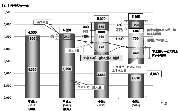
図表4-12 新たな取組による今後の総エネルギー使用量の見込み
